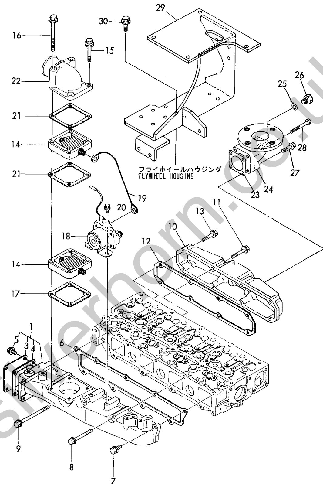
Fig. 7 吸気&排気マニホールド SUCTION & EXHAUST MANIFOLD
