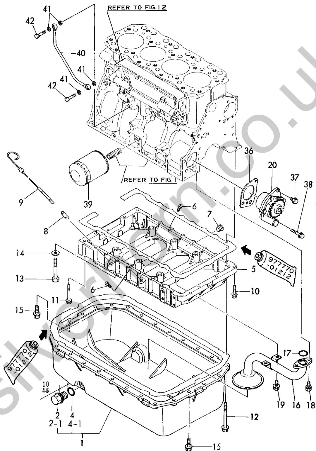
Fig. 4 潤滑油システム LUB. OIL SYSTEM
