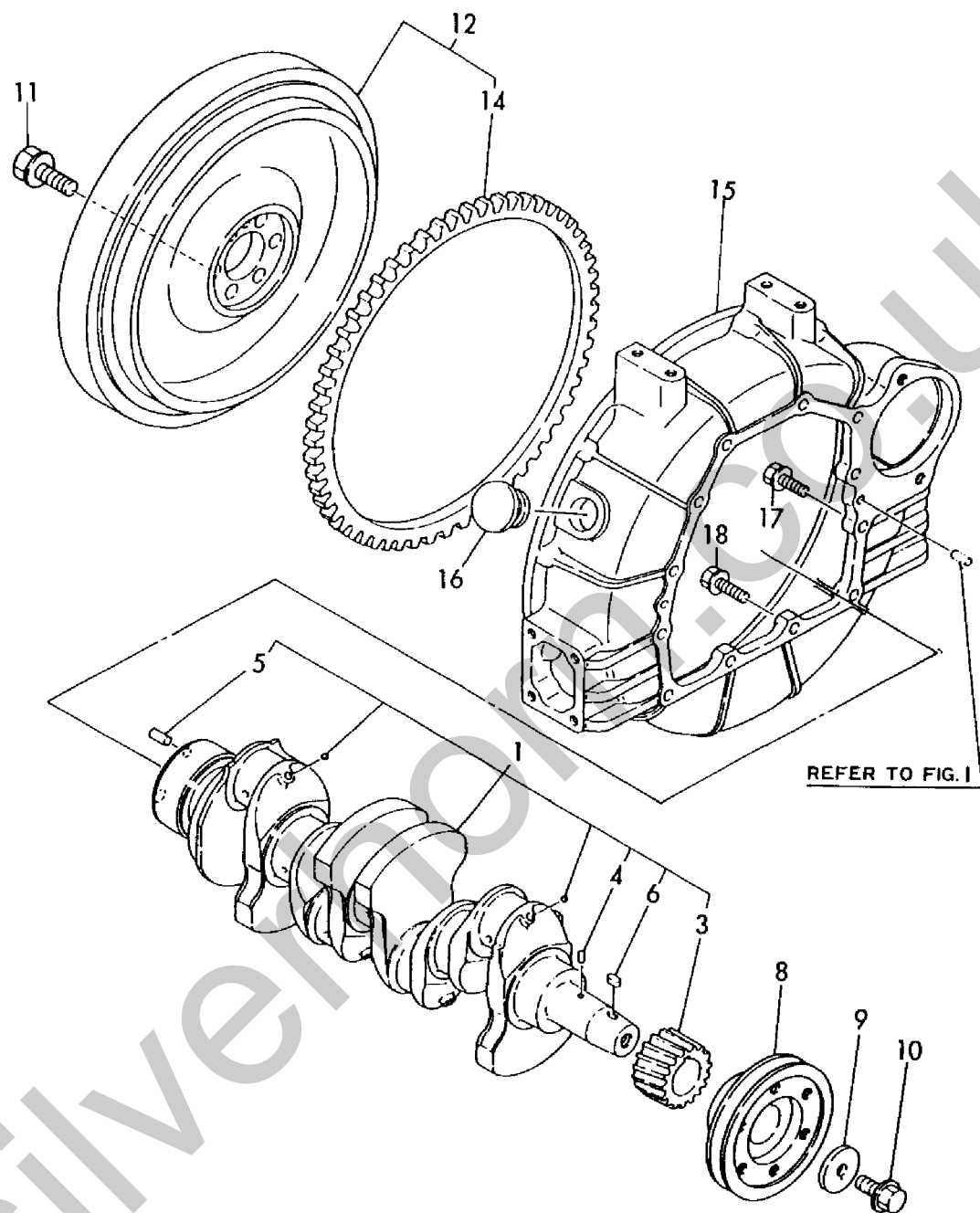
Fig. 9 クランクシャフト & フライホイール CRANKSHAFT & FLYWHEEL
