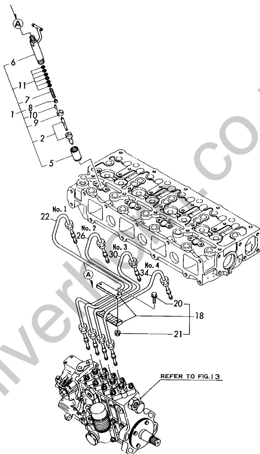
Fig. 16 燃料噴射パイプ FUEL INJECTION PIPE
