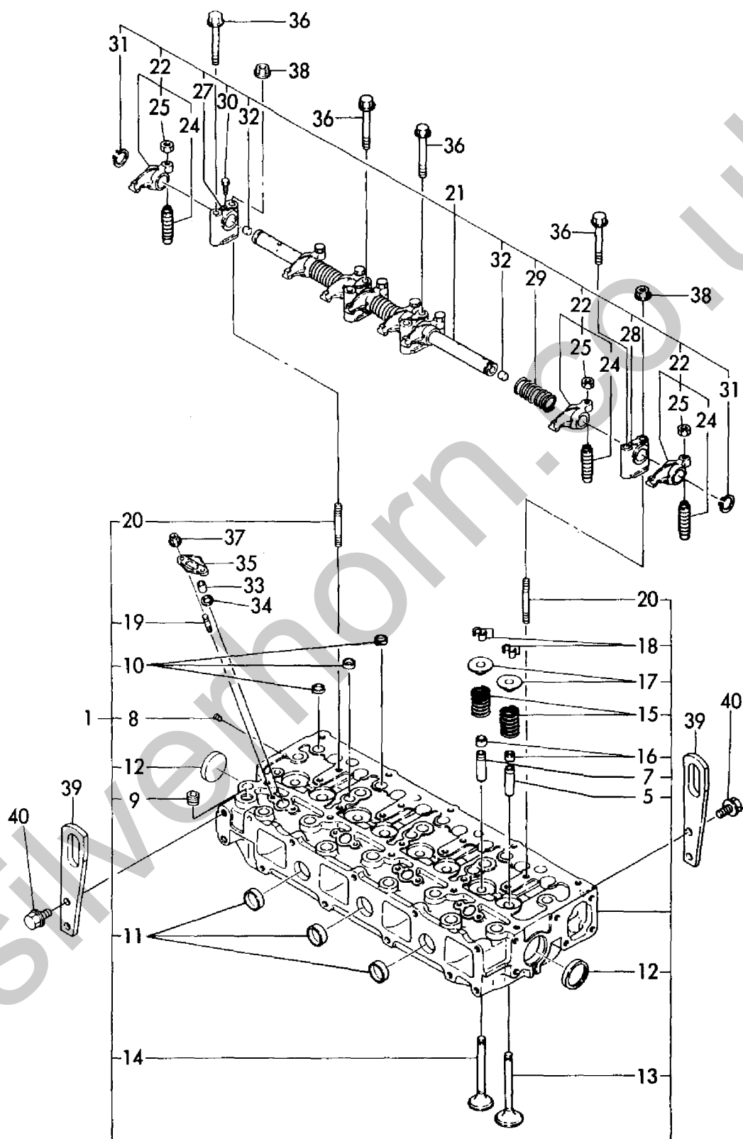
Fig. 6 シリンダヘッド CYLINDER HEAD
