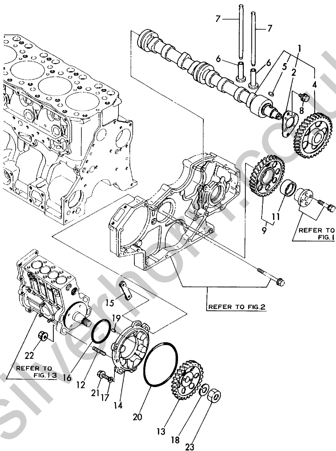
Fig. 8 カムシャフト&駆動ギヤ CAMSHAFT & DRIVING GEAR
