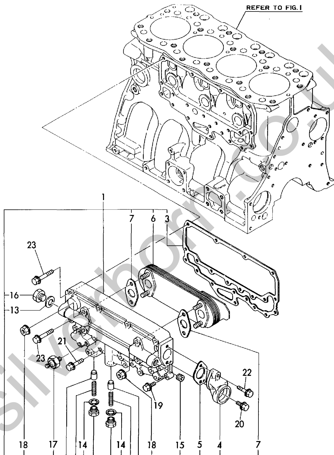
Fig. 12 オイルクーラケース OIL COOLER CASE
