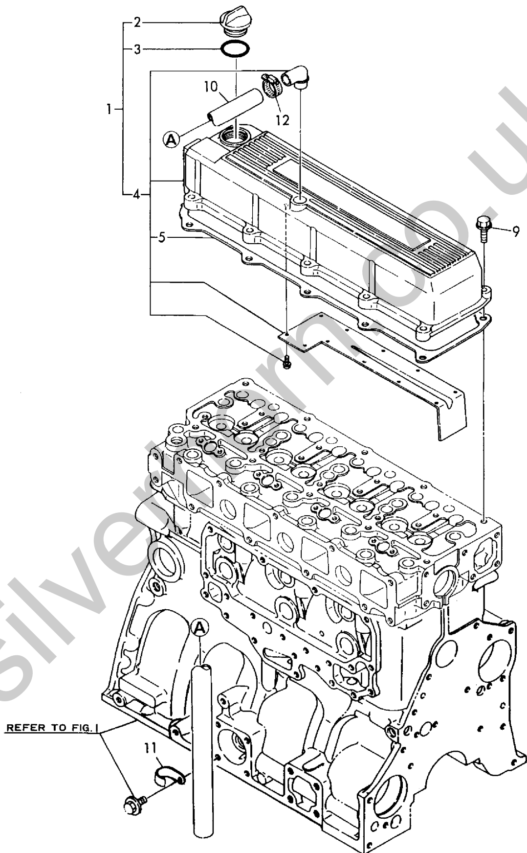
Fig. 5 ポンネット BONNET
