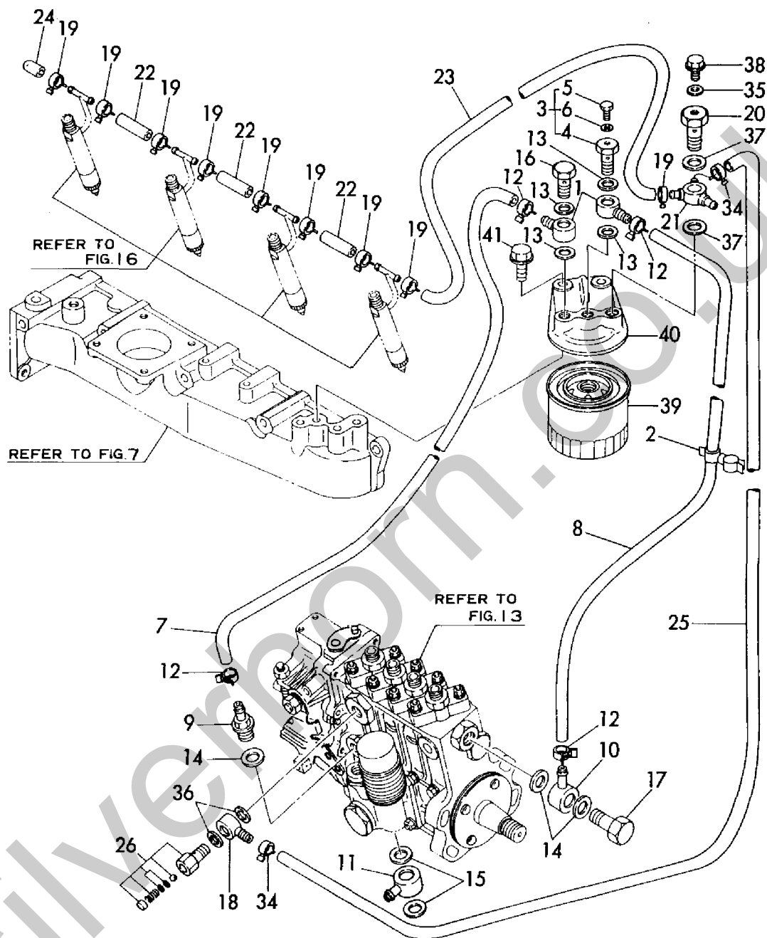
Fig. 17 燃料パイプ FUEL PIPE
