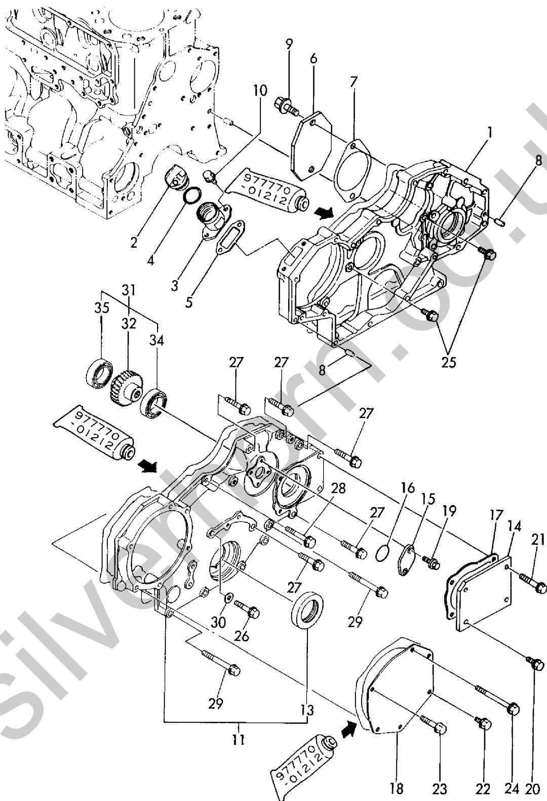
Fig. 2 ギヤケース GEAR HOUSING
