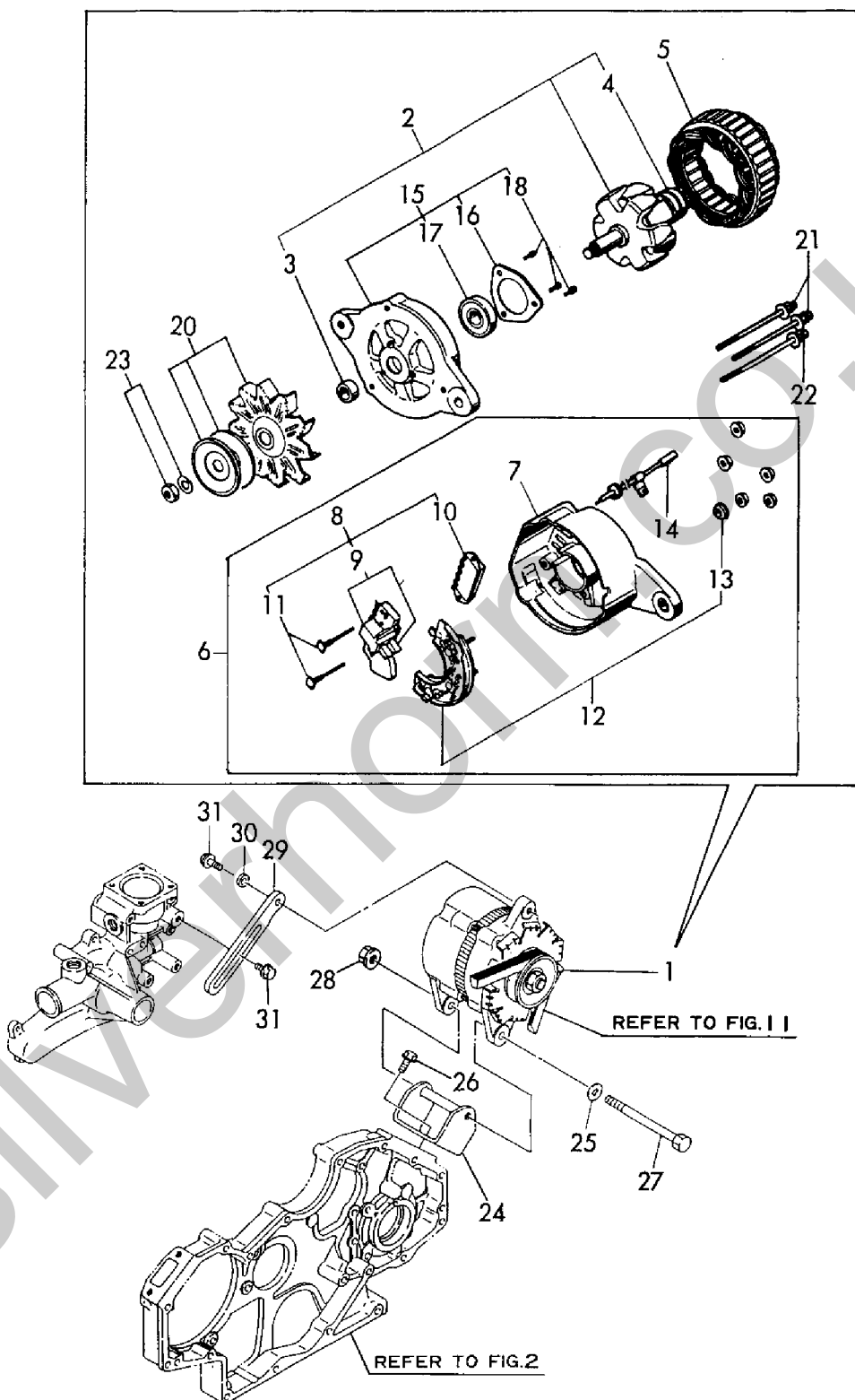
Fig. 19 ジェネレータ GENERATOR
