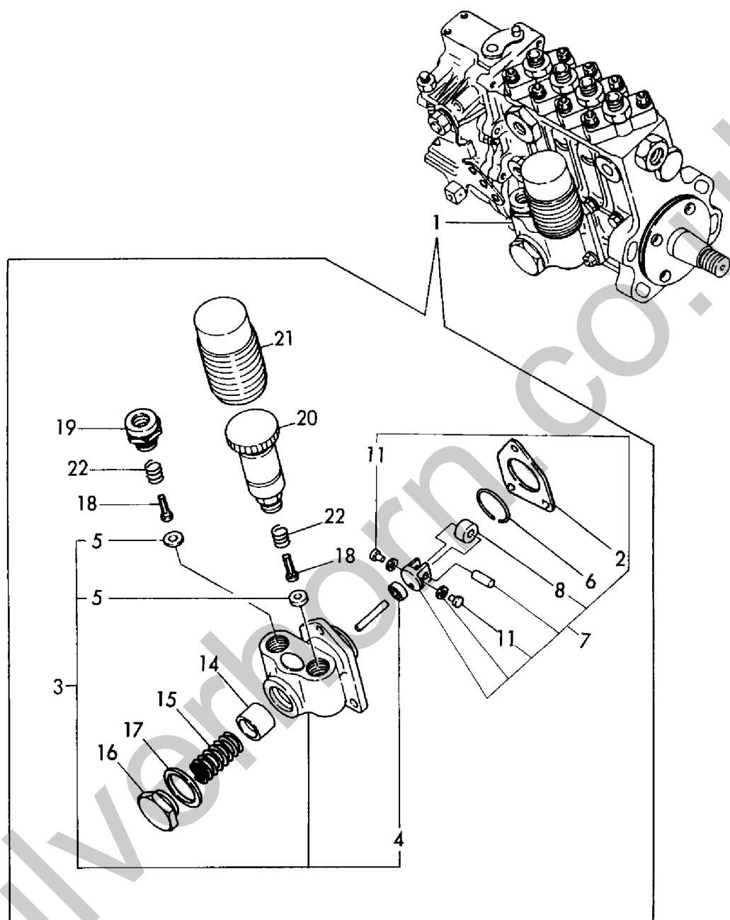
Fig. 15 フィードポンプ FEED PUMP
