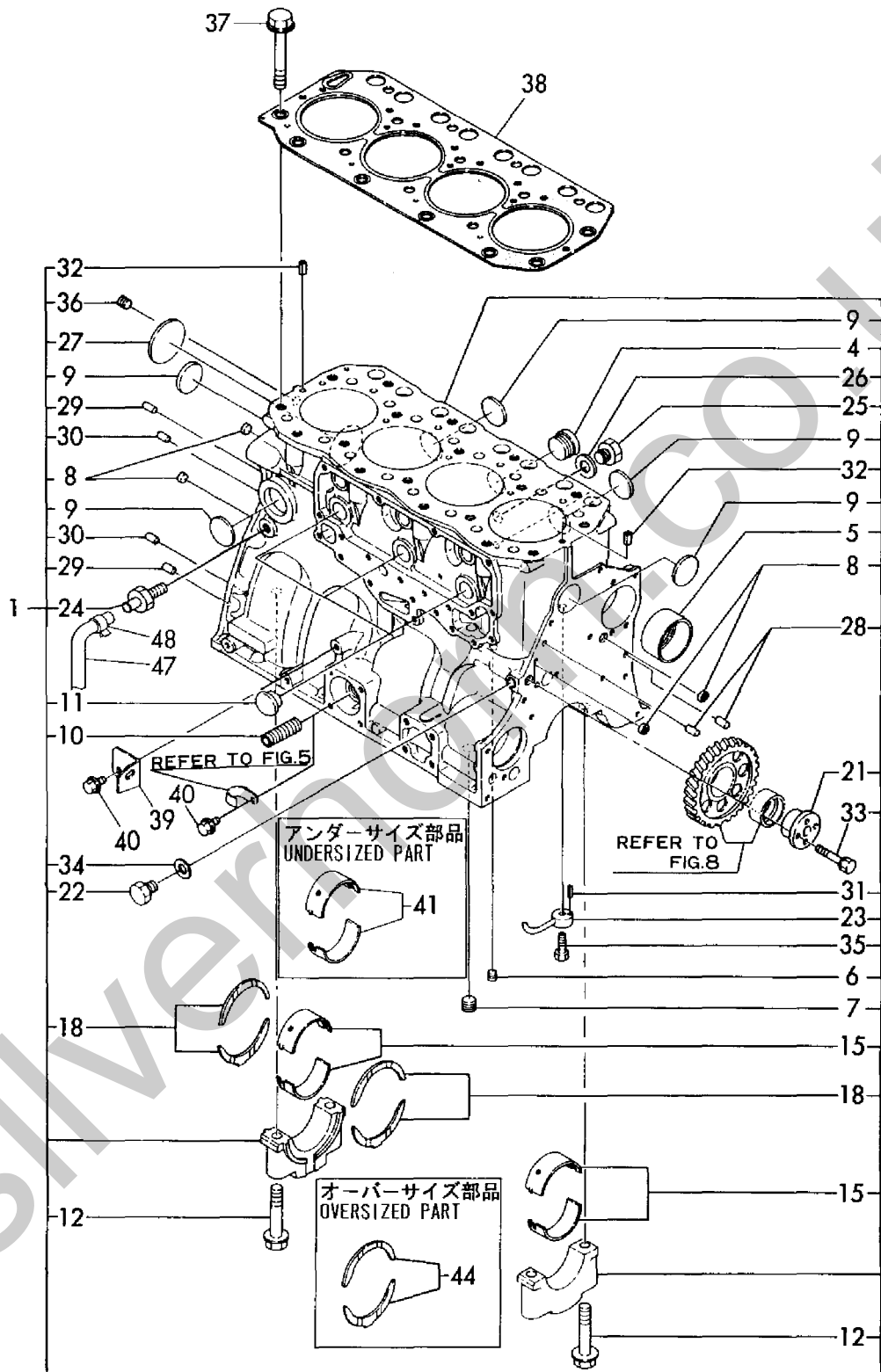
Fig. 1 シリンダブロック CYLINDER BLOCK
